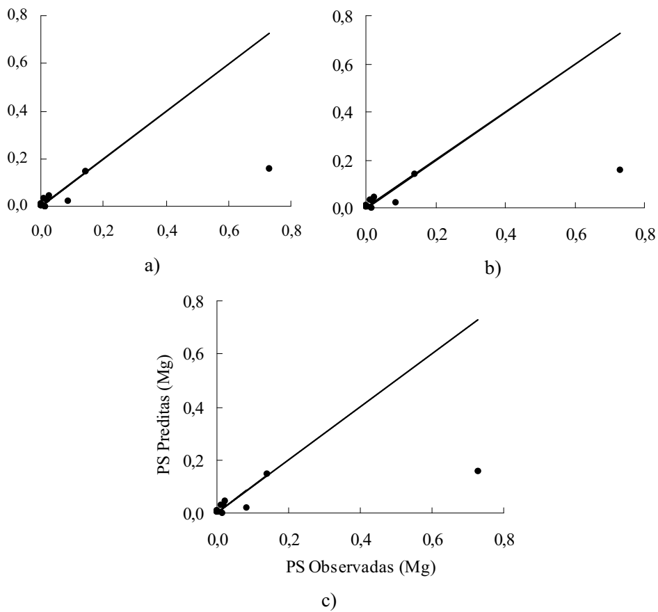
FIGURA 9 Dispersão dos valores de perdas de solo estimados pelos dados não utilizados na geração dos parâmetros “a” e “b”, por diferentes métodos de determinação do fator topográfico. a) McCool (1982); b) Paiva et al. (1995) citado por Paiva (2001); c) Williams & Berndt (1977).
