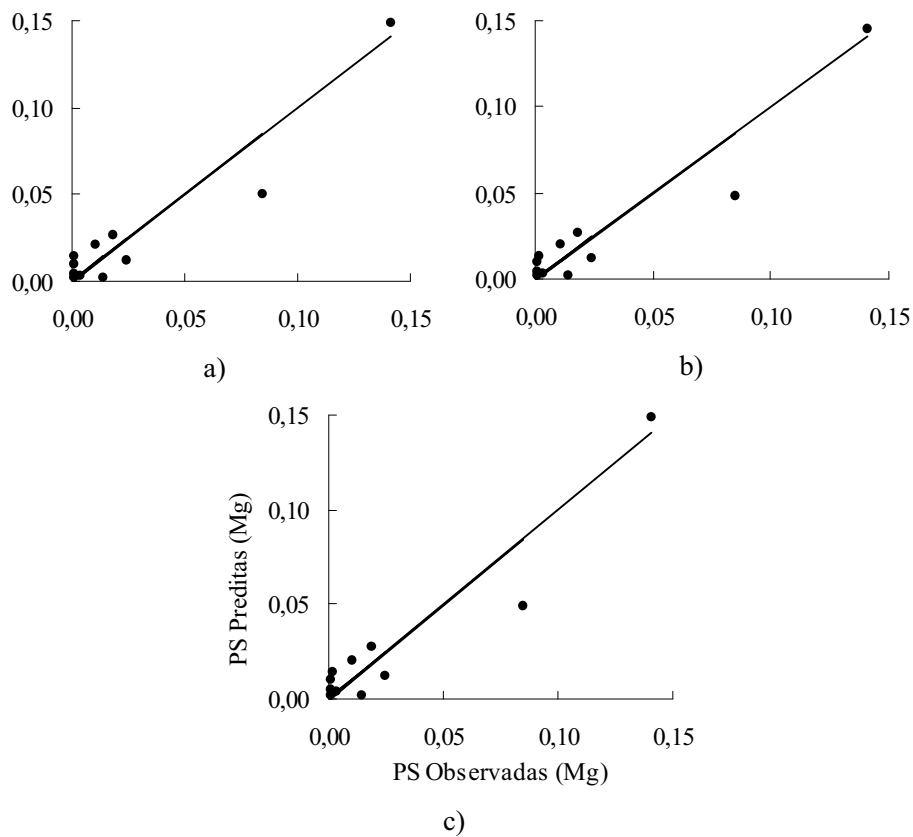
FIGURA 10 Dispersão dos valores de perdas de solo estimados pelos dados não utilizados na calibração do modelo MUSLE por diferentes métodos de determinação do fator topográfico, após exclusão do evento de precipitação do dia 02/02/2002. a) McCool (1982); b) Paiva et al. (1995) citado por Paiva (2001); c) Williams & Berndt (1977).
