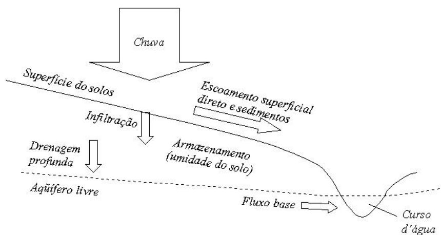
FIGURA 1 Interação entre erosão hídrica e atributos hidrológicos em uma bacia hidrográfica. Fonte: Modificado de SWCS (2003).
