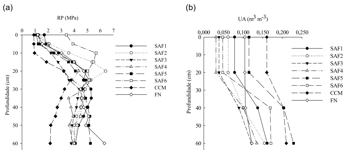
Figura 1 - (a) Resistência à penetração e (b) Umidade atual em Argissolo Amarelo típico distrocoeso, município de Prado, BA.
